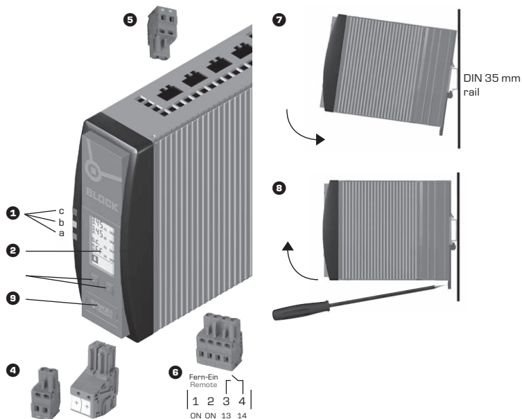
Abbildung zeigt den PVFE 24/24-40 This figure shows the PVFE 24/24-40
